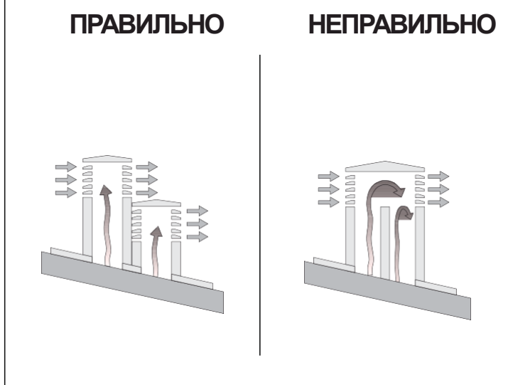
Рис. 2. Правильная установка дымохода
