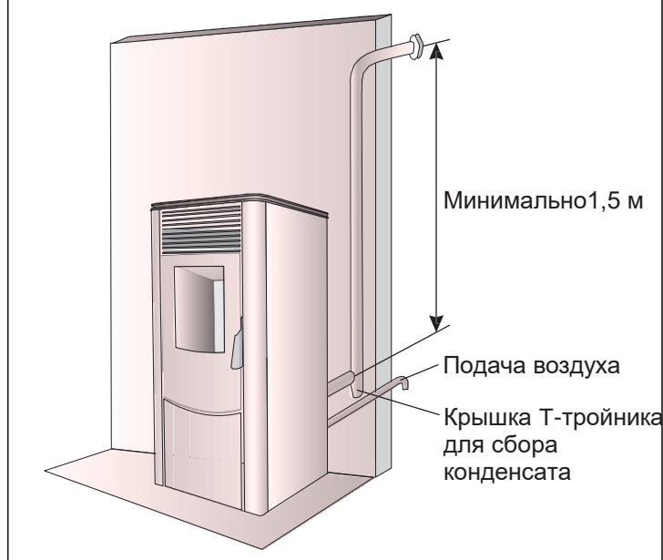
Рис. 3. Внутренняя установка дымохода, которая должна осуществляться в соответствии с правилами
