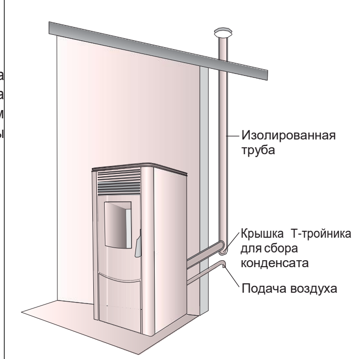
Рис. 4. Наружная установка дымохода, которая должна осуществляться в соответствии с правилами
