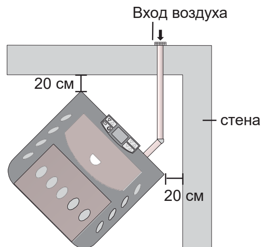
Рис. 9. Расстояние от стен
