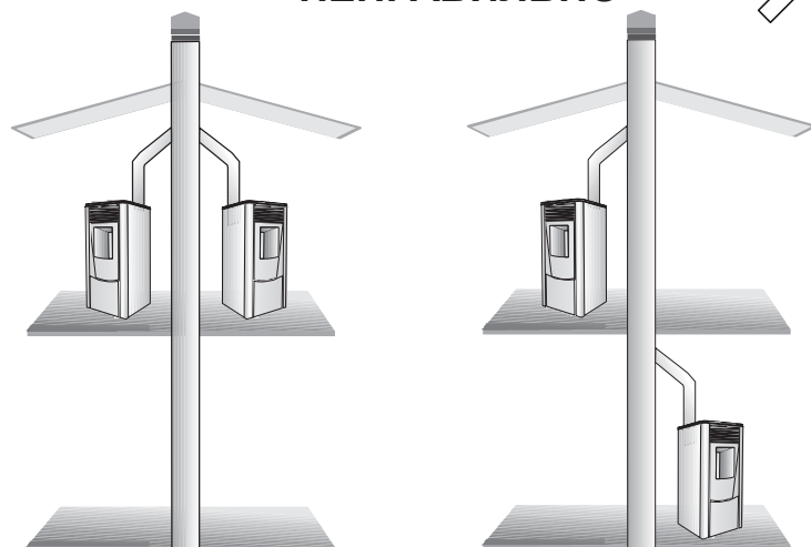
Рис. 1. Способы подключения к дымоходу
